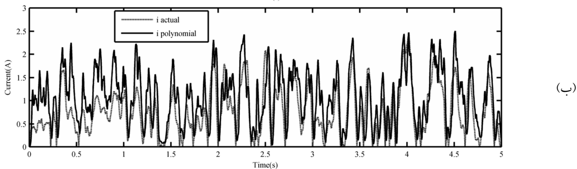
شکل ۸. مقایسه پاسخ مدل‌های میراگر در حالت معکوس با جریان واقعی (الف) مدل بوک-ون پیشنهادی، (ب) مدل چند جمله‌ای.
