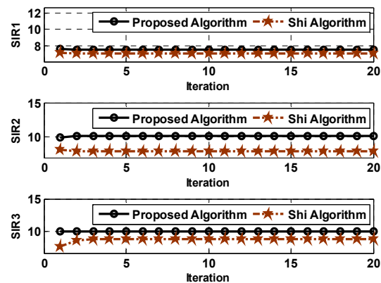
شکل ۲۰: متوسط پارامتر SNIR بازای \tau=1
