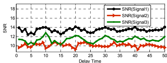
شکل ۱۰: میانگین سیگنال‌های تخمینی به‌ازای ۱۰ بار تکرار الگوریتم پیشنهادی
