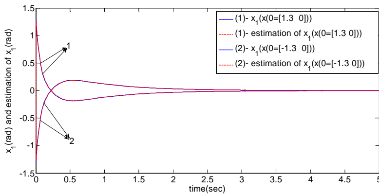
شکل ۱: پاسخ x_1(t) و تخمین آن برای مقادیر M_c = 8 و m_p = 2
