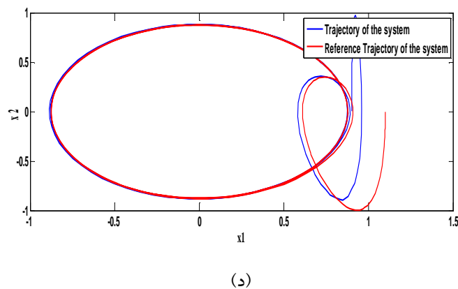
شکل ۴: الف. پاسخ زمانی متغیر حالت x_1 سیستم نوسانگر دافینگ و سیگنال مرجع برای x_1 ، ب. پاسخ زمانی متغیر حالت x_2 سیستم نوسانگر دافینگ و سیگنال مرجع برای x_2 ، ج. نیروی کنترلی و د. رفتار سیستم نوسانگر دافینگ و مدل مرجع در صفحه فاز. با توجه به شکل‌های موجود در شکل ۴ دیده می‌شود که کنترل کننده طراحی شده به خوبی توانسته است که سیستم آشوب نوسانگر دافینگ را کنترل و نتایج رضایت بخشی را ایجاد نماید. همچنین با توجه به نتایج شبیه‌سازی، محدود بودن پاسخ حالت گذرای سیستم کاملاً تضمین شده است.
