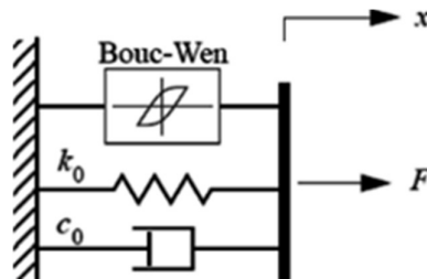
شکل ۳. مدل بوک-ون ساده [۱]
