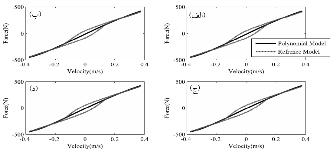
شکل ۵. مقایسه مدل چند جمله‌ای و پاسخ واقعی میراگر برای جابجایی سینوسی با دامنه 0.15 متر و فرکانس 4 هرتز (الف) جریان 0.75 آمپر، (ب) جریان 1.25 آمپر، (ج) جریان 1.75 آمپر، (د) جریان 2.25 آمپر. با توجه به شکل ۵ مشخص است که مدل چند جمله‌ای ارائه شده حلقه هیستریزیس میراگر را دنبال نکرده است. به عبارت دیگر در ناحیه سرعت پایین میراگر دقت این مدل به شدت کاهش می‌یابد. در بخش بعد دو مدل چند جمله‌ای و مدل بوک-ون ارائه شده، در حالت معکوس مورد ارزیابی قرار می‌گیرند.
