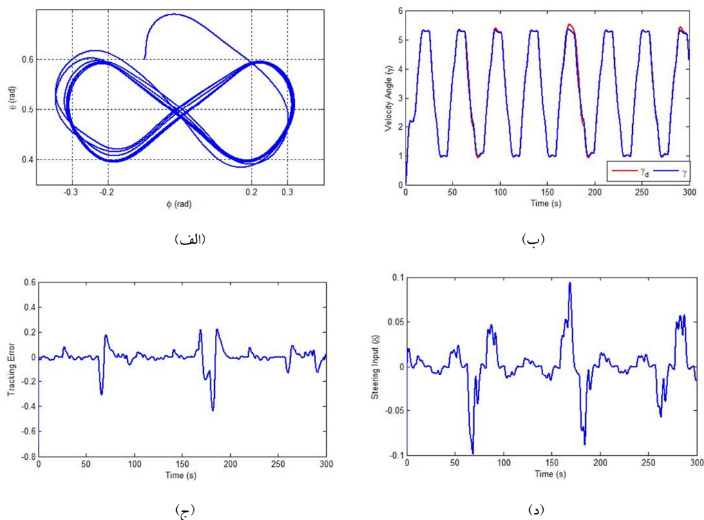
شکل ۶. (الف) مسیر حرکت سیستم در صفحه (\phi, \theta) توسط سیستم هدایتی مد لغزشی پایانه‌ای بر مبنای مسیر مطلوب تولید شده توسط نقاط هدف TP_1 و انتخاب \xi=0.5 ، \Omega=0.1 ، p=5 ، q=3 و \Delta=0.5 . (ب) نمودار زاویه بردار سرعت مطلوب (قرمز) و بردار سرعت ردیابی شده (آبی)، (ج) نمودار خطای ردیابی زاویه بردار سرعت بر حسب زمان، (د) نمودار ورودی هدایتی ( \delta ) تولید شده توسط کنترل کننده.
