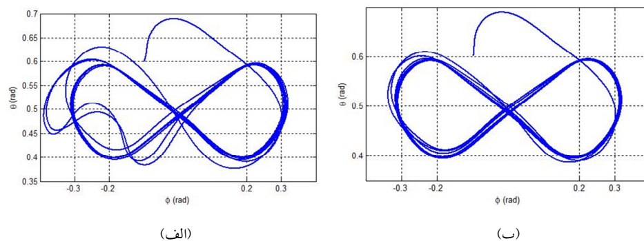
شکل ۷. مسیر حرکت در صفحه (\phi, \theta) توسط سیستم هدایتی مد لغزشی پایانه‌ای بر مبنای مسیر مطلوب برای نقاط هدف TP_1 و (الف) \xi=0.3 ، \Omega=0.1 ، p=5 ، q=3 و \Delta=0.5 ، (ب) \xi=0.7 ، \Omega=0.1 ، p=5 ، q=3 و \Delta=0.5 . پارامتر بعدی که مورد بررسی قرار می‌گیرد پارامتر \Omega می‌باشد. این پارامتر با زمان حذف انحراف از مقدار مطلوب ( T_{dyn} ) نسبت عکس دارد و مقادیر بزرگ‌تر آن این زمان را کاهش می‌دهد. تصویر ۸ نتایج شبیه‌سازی برای مسیر ردیابی شده توسط سیستم را در دو حالت با \Omega مختلف نشان می‌دهد.
