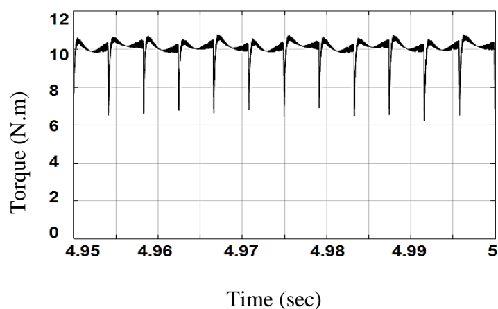
شکل (۲۲). شکل موج تغییرات گشتاور الکترومغناطیسی موتور BLDC
