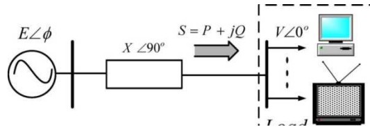
شکل ۱: مدار معادل تکفاز اینورتر متصل به بار
