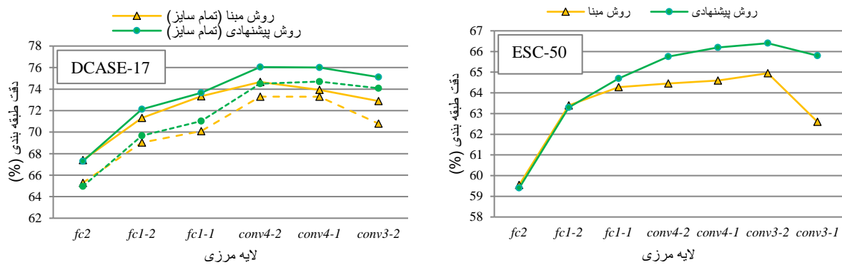
شکل ۵- میانگین دقت های طبقه بندی حاصل از تطبیق شبکه به روش مینا و روش پیشنهادی به روی بخش توسعه دادگان DCASE-17 (به ازای آموزش با تمام دادگان آموزش و نیمه از آن) و میانگین دقت های حاصل از اعتبارسنجی ارائه شده در [12].
