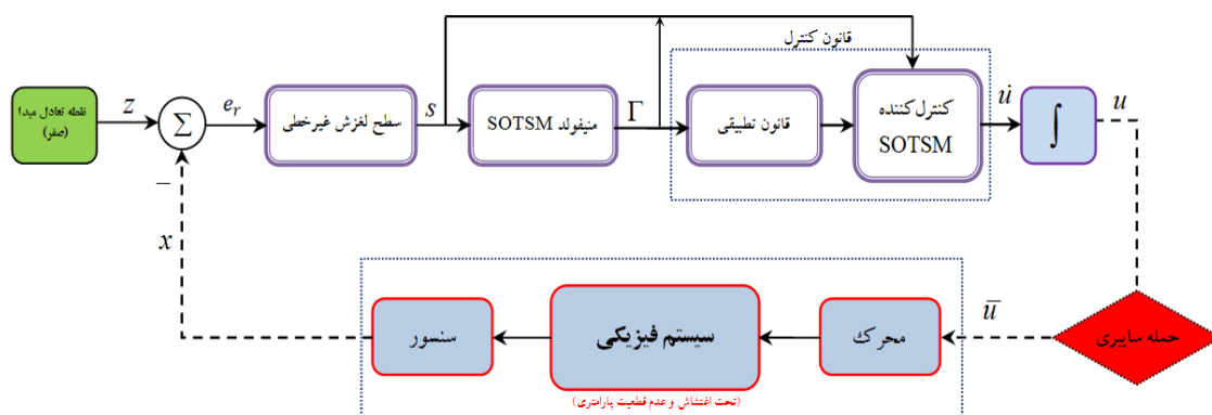
شکل ۲- شماتیک کنترل کننده SOTSM تطبیقی طراحی شده برای سیستم های فیزیکی سایبری در حضور عدم قطعیت پارامتری، اغتشاش ناخواسته و حمله سایبری محرک
