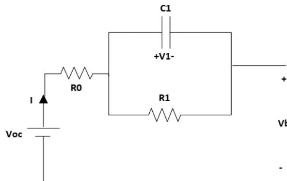
شکل ۱- مدل مرتبه اول باتری
