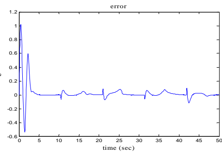
شکل ۱۳: اختلاف خروجی فرایند و خروجی مدل مرجع
