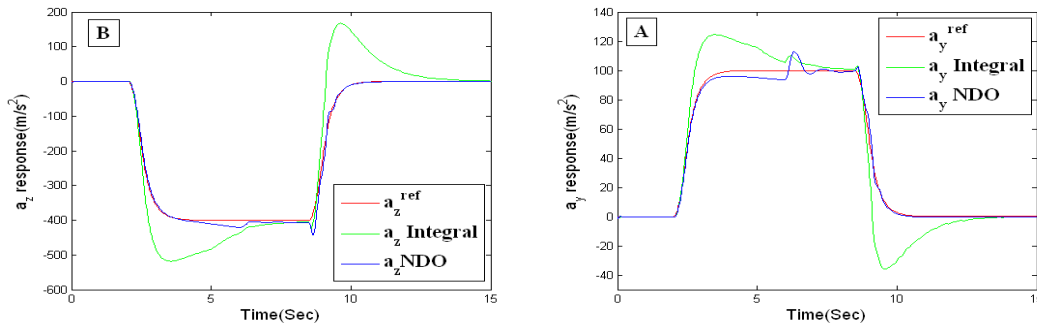
شکل ۱۰: مقایسه‌ی عملکرد کنترل کننده‌ی تطبیقی- لغزشی همراه با NDO با عملکرد کنترل کننده‌ی مبتنی بر تکنیک گام به عقب بهبود یافته همراه با انتگرالگیر در ردیابی سیگنال‌های شتاب مرجع؛ (A) ردیابی سیگنال شتاب a_y و (B) ردیابی سیگنال شتاب a_z . (عنوان انتگرال برای روش گام به عقب بهبود یافته ی مرجع [۷] ذکر شده است).
