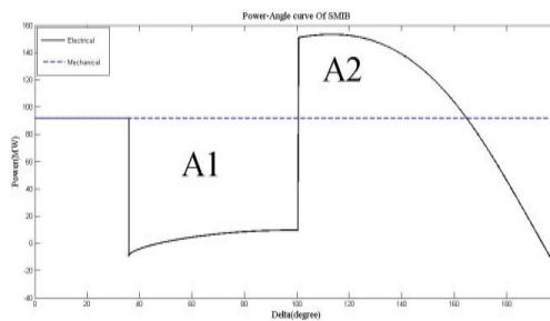
شکل ۲۲: منحنی توان-زاویه ماشین معادل شبکه
