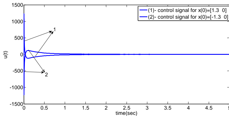
شکل ۵: سیگنال کنترلی u(t) برای m_p = 2 و M_c = 8
